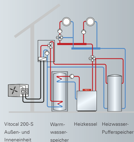
Vitocal 200-S und Öl-/Gas-Heizkessel für den bivalenten Betrieb bei der Modernisierung (Anlagenbeispiel: AWB)
