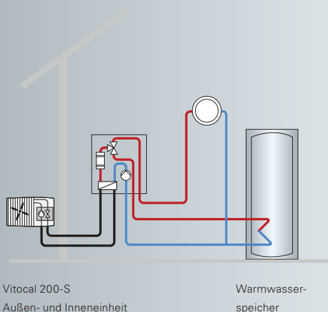
Vitocal 200-S als Heizungssystem im Neubau (Anlagenbeispiel: AWB-AC)
