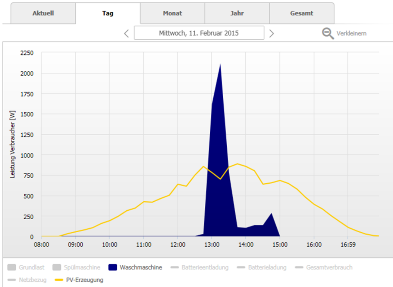
Abbildung 7: Darstellung auf der Seite Verbraucherbilanz und -steuerung (Beispiel)
