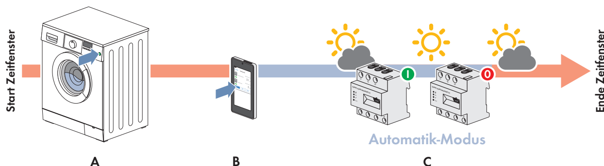
Abbildung 6: Ablauf der Verbrauchersteuerung über den Sunny Home Manager
