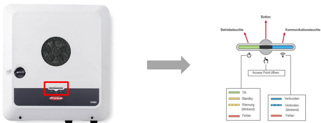
Abbildung 9: Öffnen des lokalen Netzwerkes (Wifi-Access Point) der Fronius GEN24 Plus Wechselrichterserie und Beschreibung der Funktionen der LED-Muster
